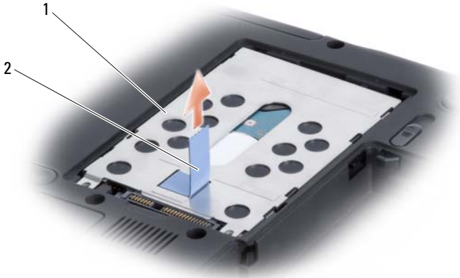
1 하드 드라이브 조립품 2 당김 탭
