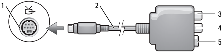
1 S-video TV-out 커넥터
